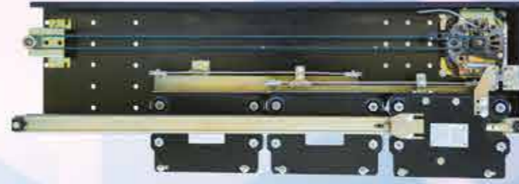
Teleskopik 3 Panel İnce Seri Kabin Operatörü Slim Series 3 Panels Telescopic Car Door Operator Opérateur de Porte Cabine Téléscopique, 3 Vantaux, Série Slim
